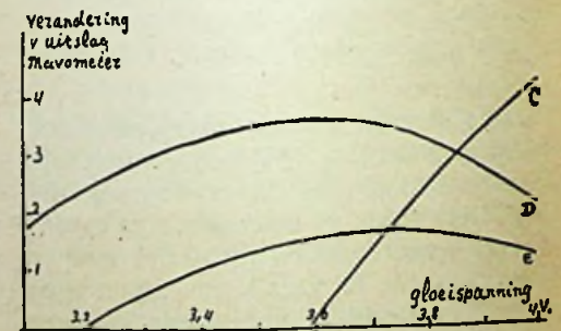
Fig. 2. Afhankelijkheid der ijking van de gloei-spanning bij constante roosterwisselspanning (C, D en E als in fig. 1).
