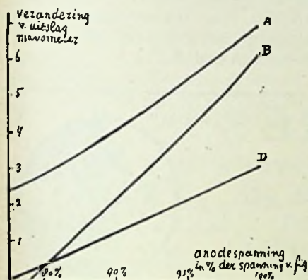
Fig. 3. Afhankelijkheid der ijking van de anodespanning bij constante roosterwisselspanning. (A, B en D als in fig. 1).
